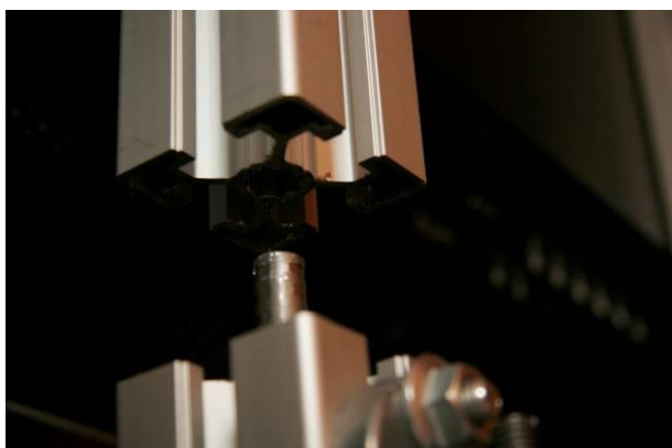
Стыковка верхней и нижней панелей
