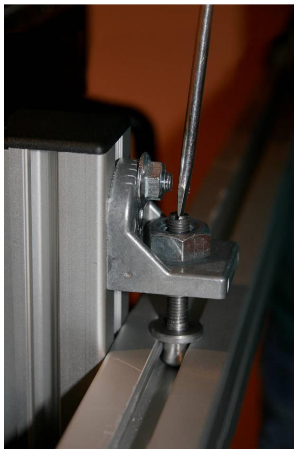
Регулирование вертикального расположения панели
